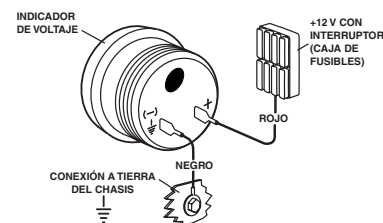
Figura 4. Conexiones de Voltímetro
